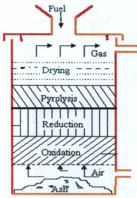
ภาพที่ 6.9 ระบบผลิตก๊าซเชื้อเพลิงแบบไหลขึ้น (Updraft Gasifier)
