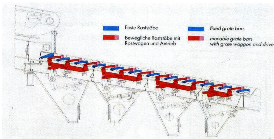
ภาพที่ 6.3 ส่วนประกอบของตะกรับที่ช่วยให้มูลฝอยเกิดการเคลื่อนที่
