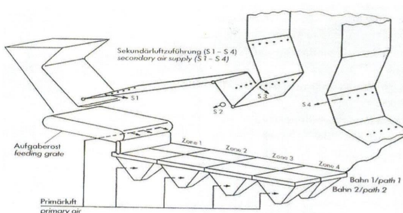
รูปที่ 6.4 อากาศที่ใช้ในการเผาไหม้ที่จ่ายเข้าตามส่วนต่าง ๆ ของห้องเผาไหม้
