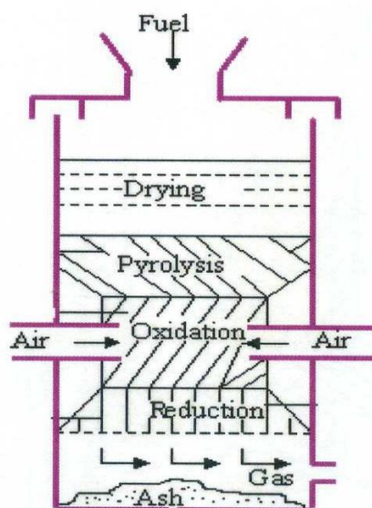
รูปที่ 6.10 ระบบผลิตก๊าซเชื้อเพลิงแบบไหลลง (Downdraft gasifier) ที่มา : http://biofuelsacademy.org
