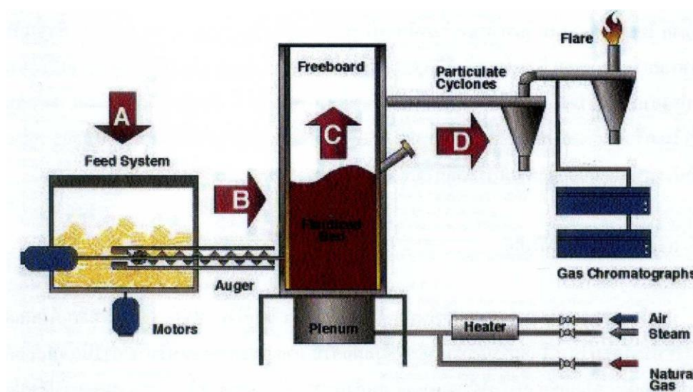
ภาพที่ 6.12 ระบบผลิตก๊าซเชื้อเพลิงแบบป้อนเชื้อเพลิงต่อเนื่อง (Fluid Bed Gasifier)
