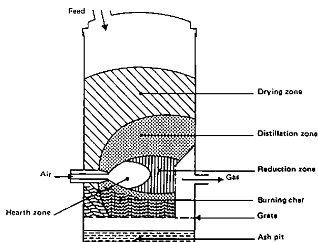
รูปที่ 6.11 เครื่องปฏิกรณ์แก๊สซิฟายเออร์แบบไหลขวาง (cross draft gasifier)
